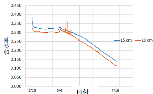
図5 含水率変化 (電気抵抗センサによる)
