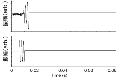
図7 6/18 送信周波数700 Hzにおける 上：受信波形 下：送信波形 (深度25 cm 根有り経路 伝搬距離23 cm)
