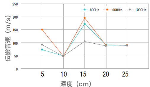
図10 送信周波数800、900、1000 Hzにおける 深度ごとの伝搬音速
