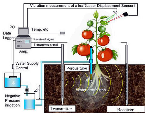
図1 実験構想図
