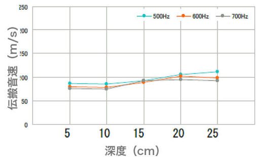
図9 送信周波数500、600、700 Hzにおける 深度ごとの伝搬音速
