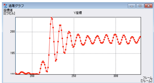
Fig.9 P2 特徴点追尾結果例
