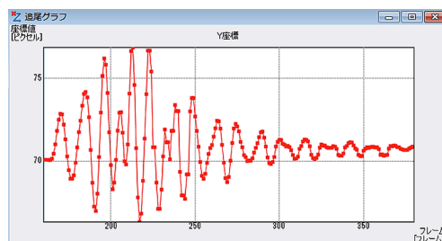
Fig.6 P1 特徴点追尾結果例
