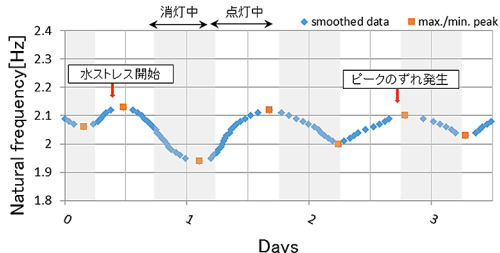
Fig.1 固有振動数連続計測結果例
